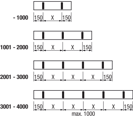
VA3100 Hide Disposizione e numero di supporti di fissaggio / fori
