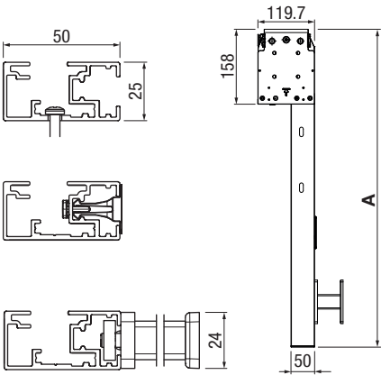
VA3100 Hide Guida a 1 pezzo VA110
