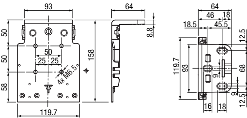
VA3100 Hide Console a soffitto / pavimento VA310
