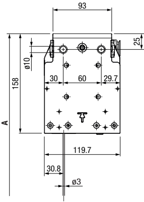
VA3100 Hide Montaggio con guida per cavi
