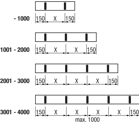
VA3100 Hide Disposition et nombre de supports de fixation / per ages
