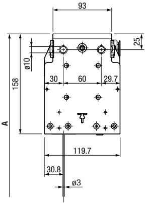
VA3100 Hide Montage avec guide-câble
