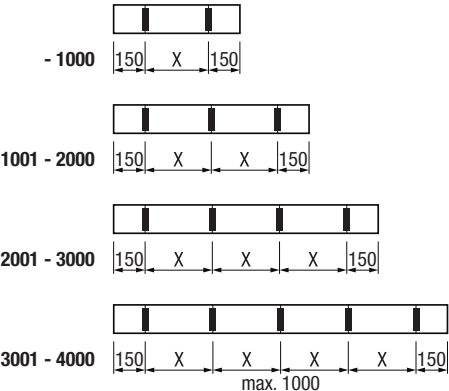
VA3100 Hide Anordnung und Anzahl Befestigungshalter / Stanzungen
