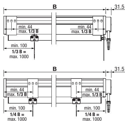
Ingesprongen draadgeleiding
