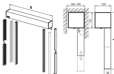
Gedeelde, 2-delige geleiderail
