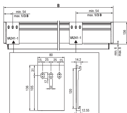
Montage met wandconsole
