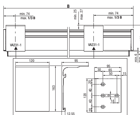
Montage met plafondconsole
