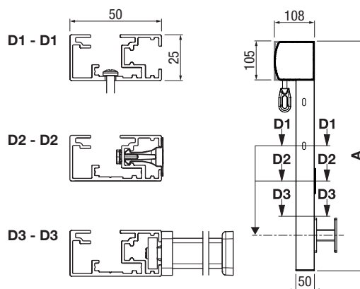
Opzetmontage 1-delige geleidingsrail VA110
