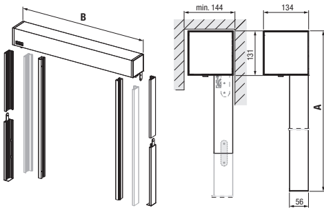
VA2300 Box Rail de guidage divisé en deux parties
