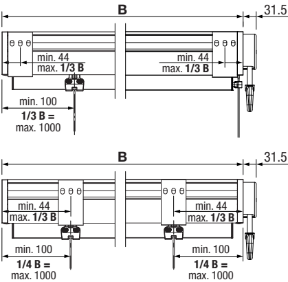
VA2100 Box Guide-câble encastré
