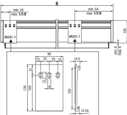
VA2300 Box Montage avec console murale
