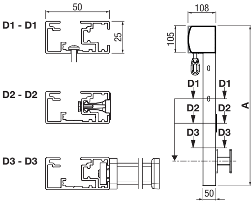
VA2100 Box Montage par emboîtement Coulisse en 1 partie VA110
