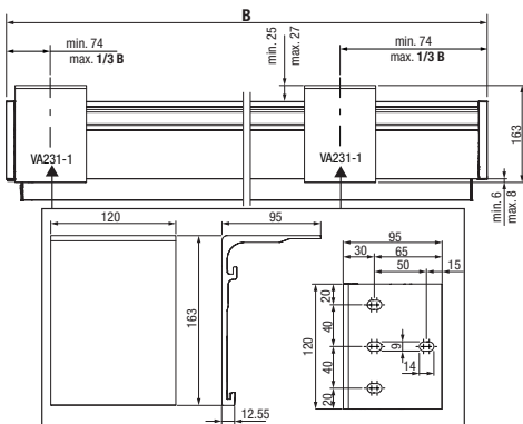
VA2300 Box Montage avec console sous dalle
