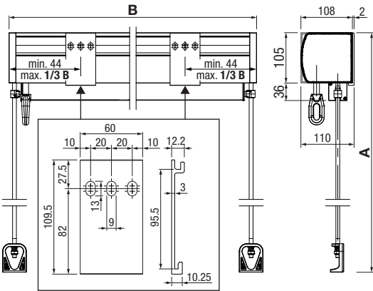
VA2100 Box Montage avec console murale
