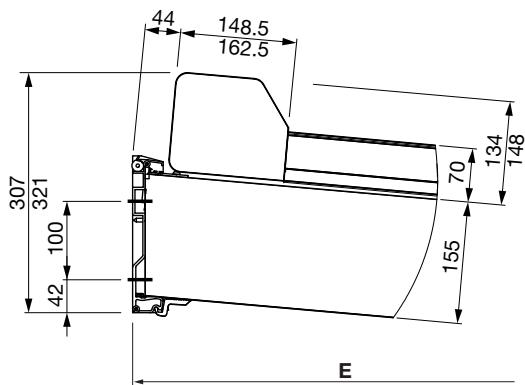
GP3100 Wandaansluiting
