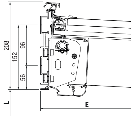
GP4100 Collegamento a parete
