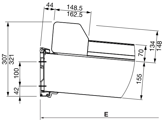
GP3100 Collegamento a parete
