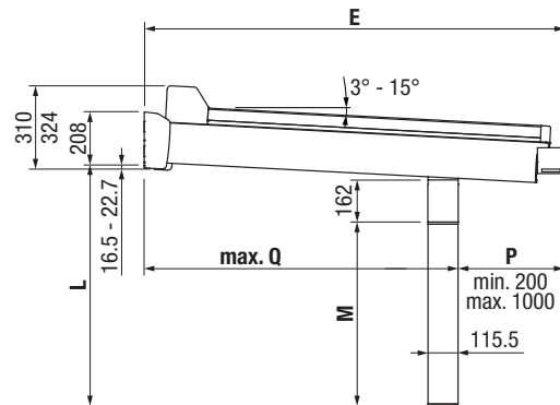
GP4200 Vista laterale
