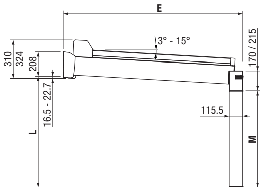
GP4100 Vista laterale
