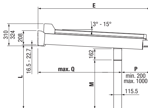
GP4200 Vue latérale
