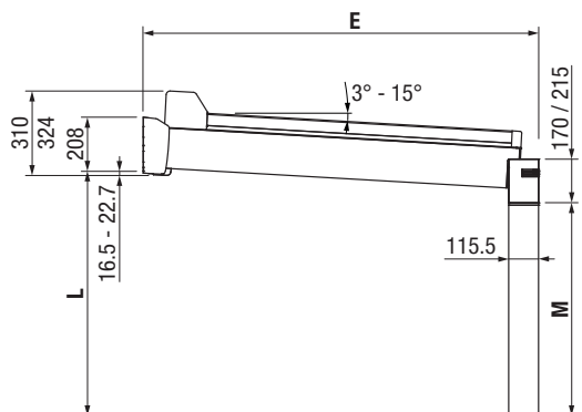
GP4100 Vue latérale
