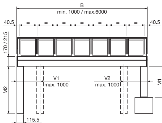
GP3100 Vue frontale
