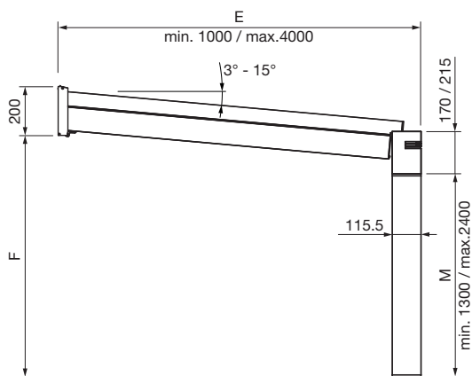
GP3100 Vue latérale
