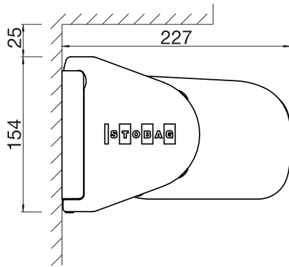
BX2000 Wandmontage Ausfallprofil abgerundet
