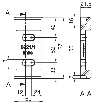
BX2000 S721/1 Konsole
