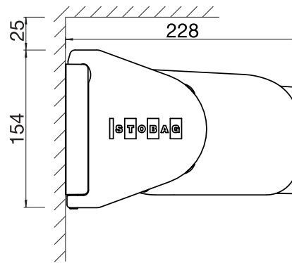
BX2000 Wandmontage mit eckigem Ausfallprofil
