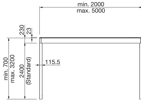
TP6100 Frontansicht
