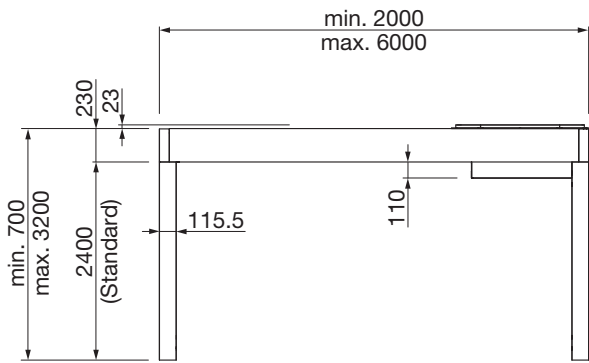
TP6100 Seitenansicht
