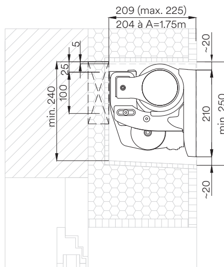
Coupe d'une variante de montage et de niche, angle d'inclinaison 0° – 5°, façade crépie
