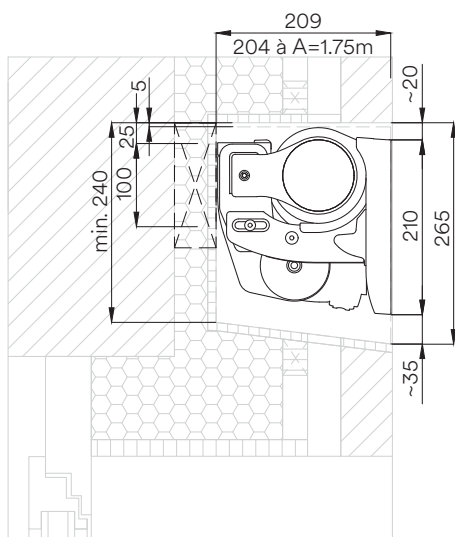
Coupe d'une variante encastrée et en niche, angle d'inclinaison 5° – 10°, façade ventilée
