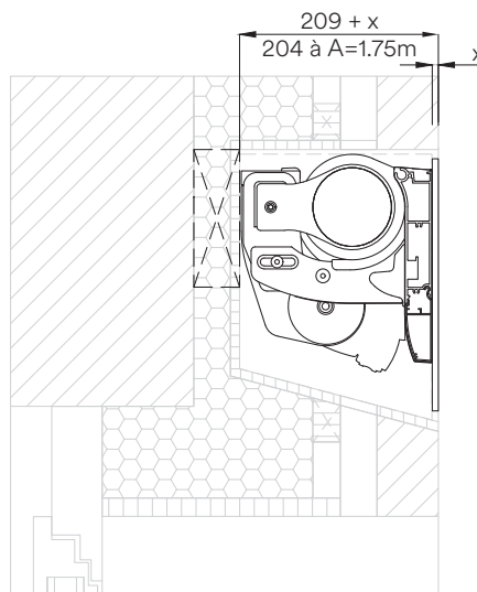
Coupe Montage du bandeau par le client, angle d'inclinaison 15° – 20°, façade ventilée
