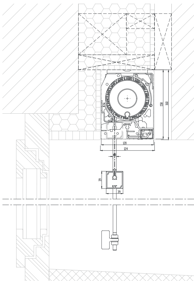
Montage au plafond avec guidage par tige, coupe d'une variante encastrée et en niche
